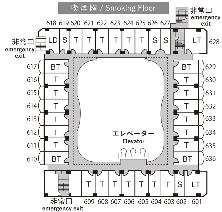
《 6階客室平面図 / 6th Floor 》
