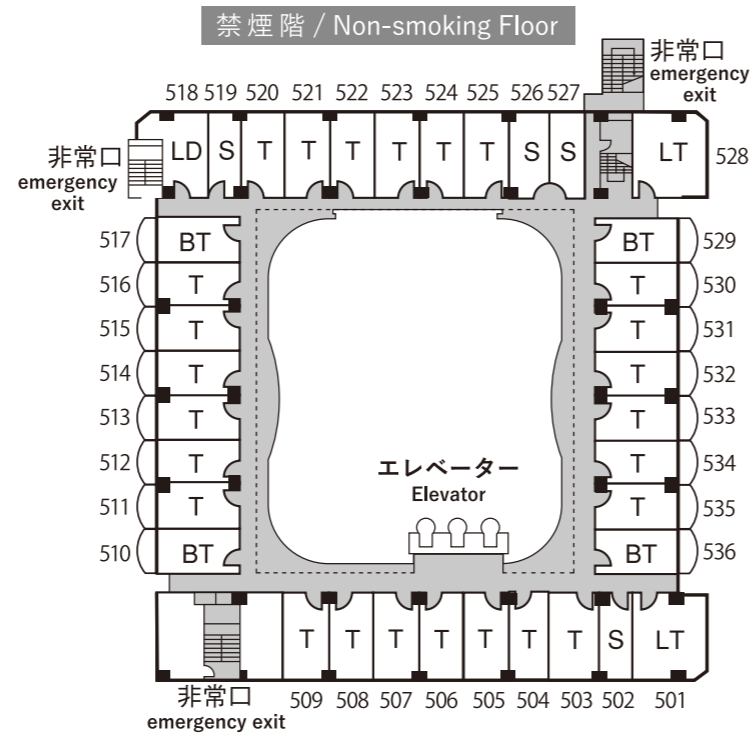
《 5階客室平面図 / 5th Floor 》
