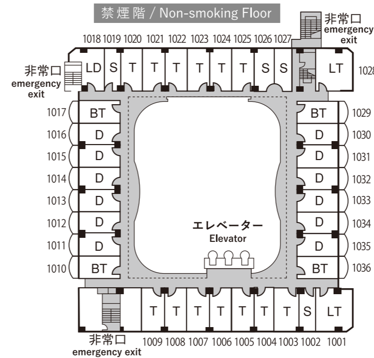
《 10階客室平面図 / 10th Floor 》
